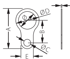
Uchwyt uziemienia
